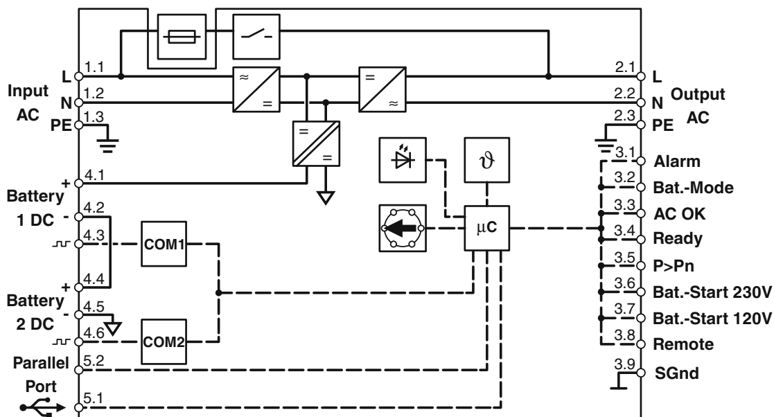
Schemat blokowy
