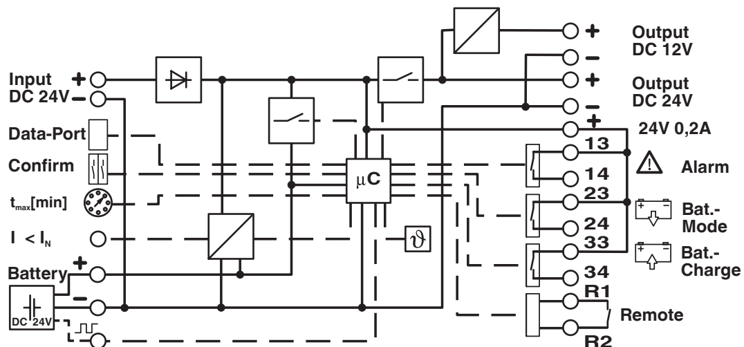
Schemat blokowy
