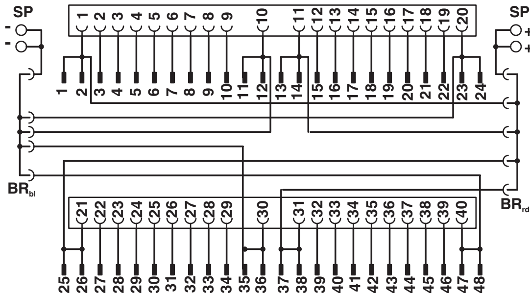
Schemat
