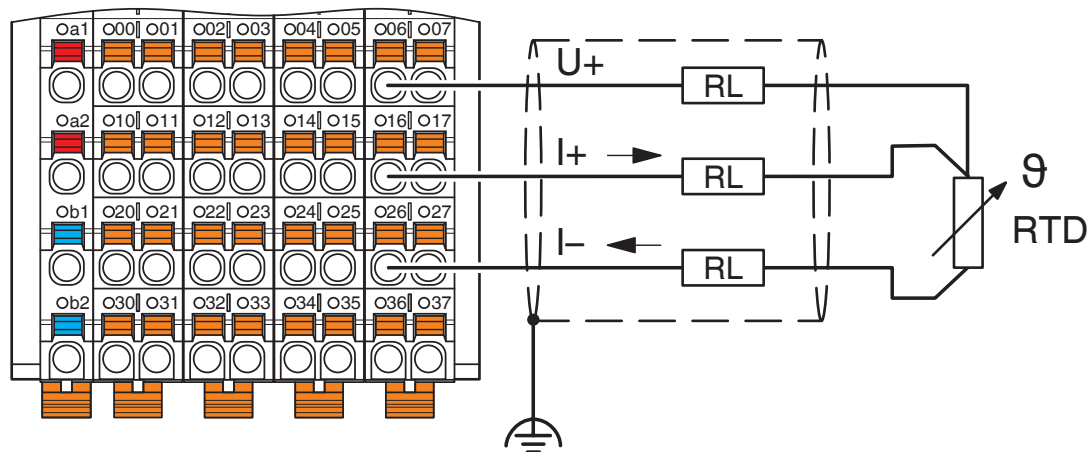
rysunek złączy
