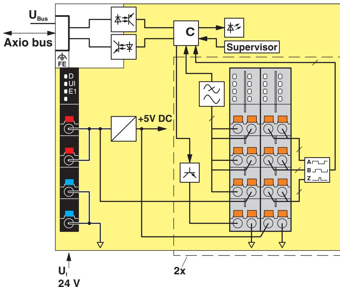
Schemat blokowy
