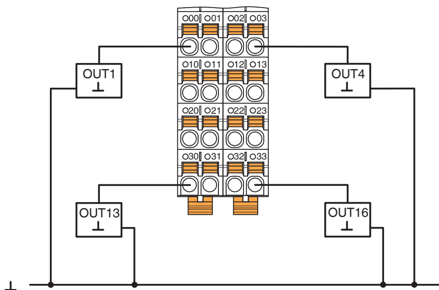
rysunek złączy
