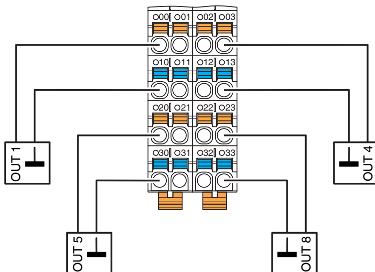
rysunek złączy
