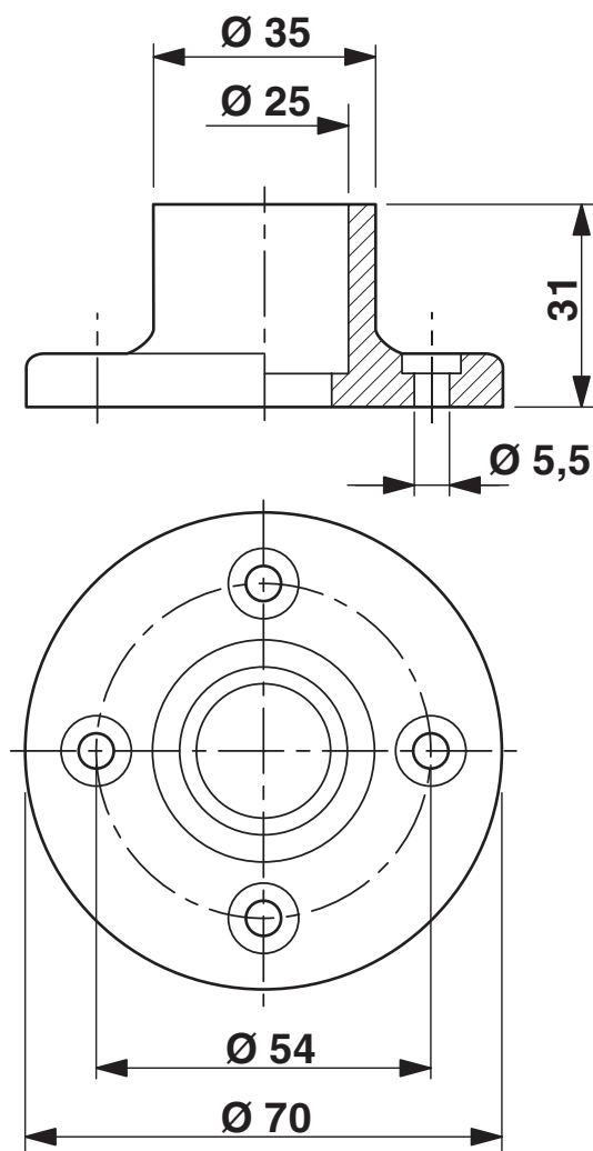
Rysunek wymiarowy
