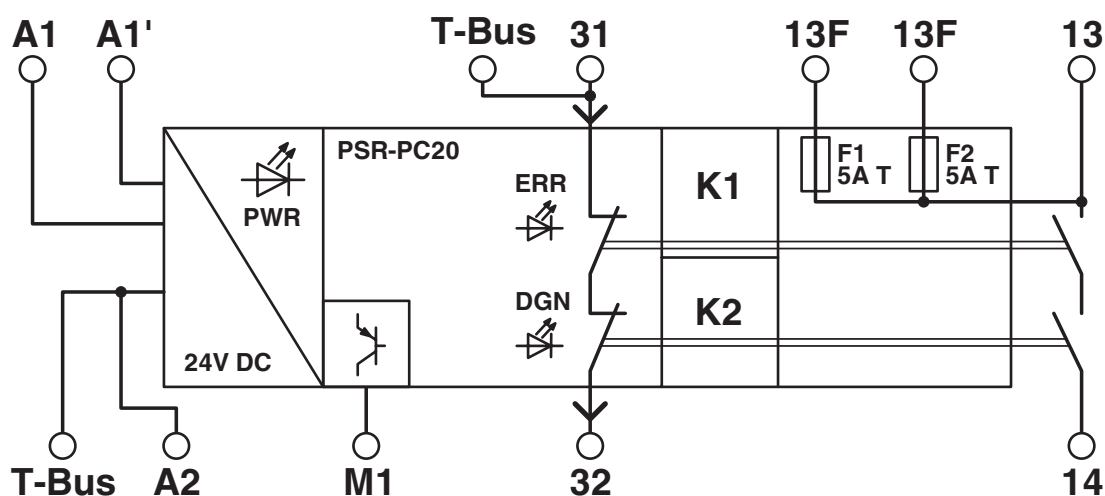
Schemat blokowy
