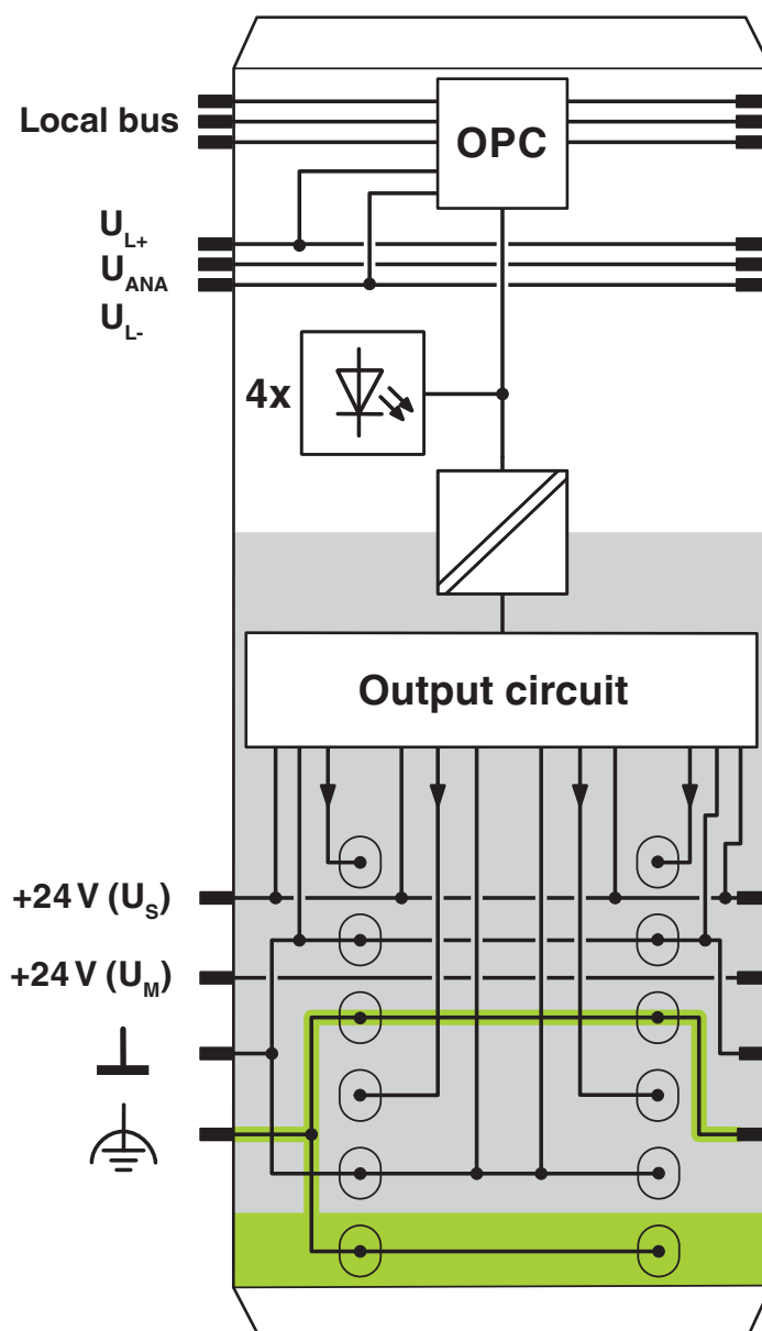
Schemat blokowy
