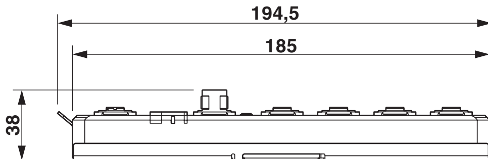
Rysunek wymiarowy
