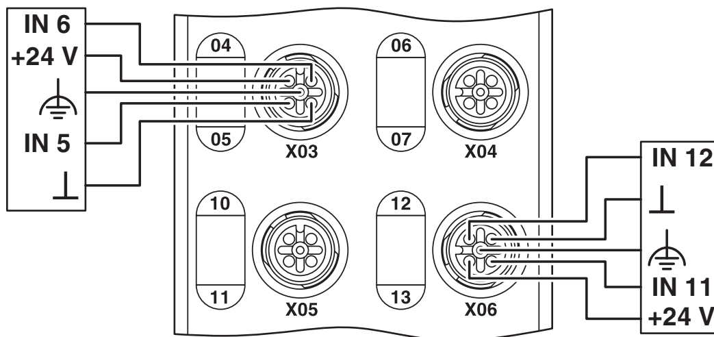
rysunek złączy
