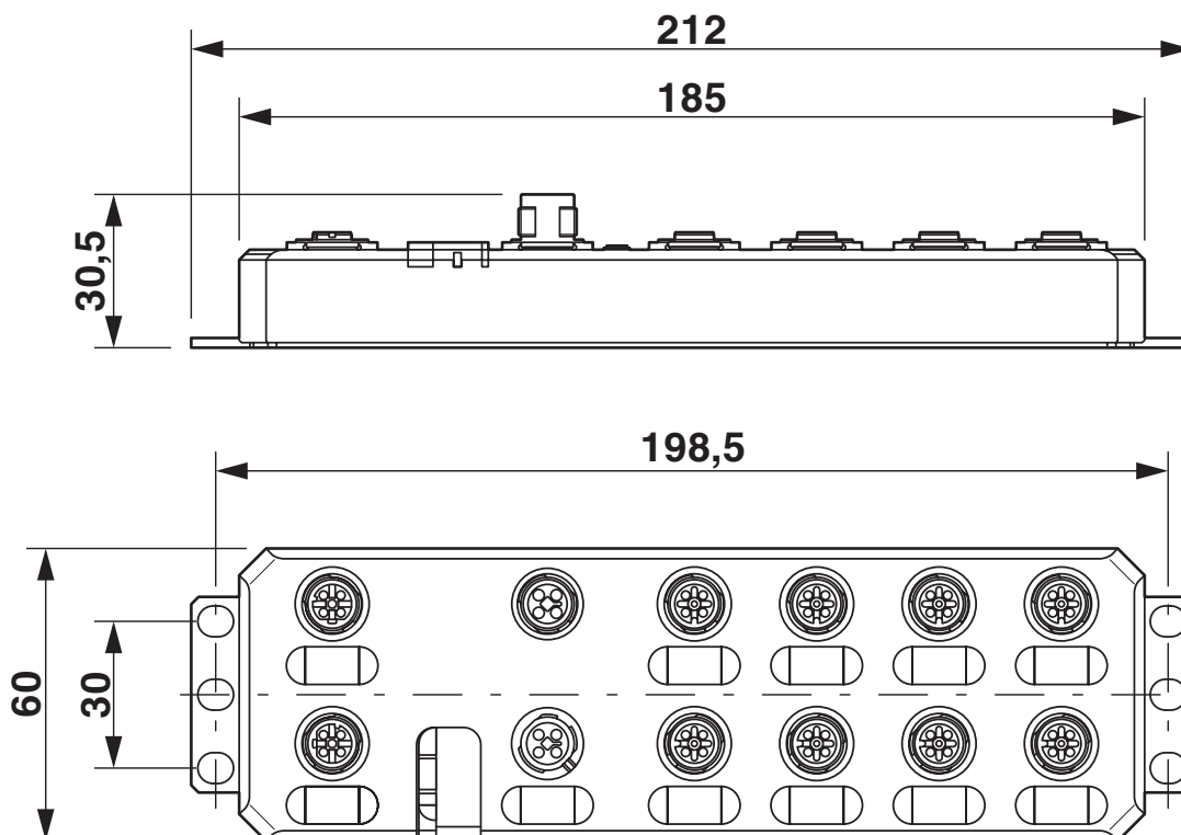
Rysunek wymiarowy
