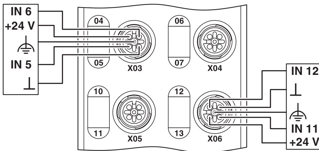
rysunek złączy
