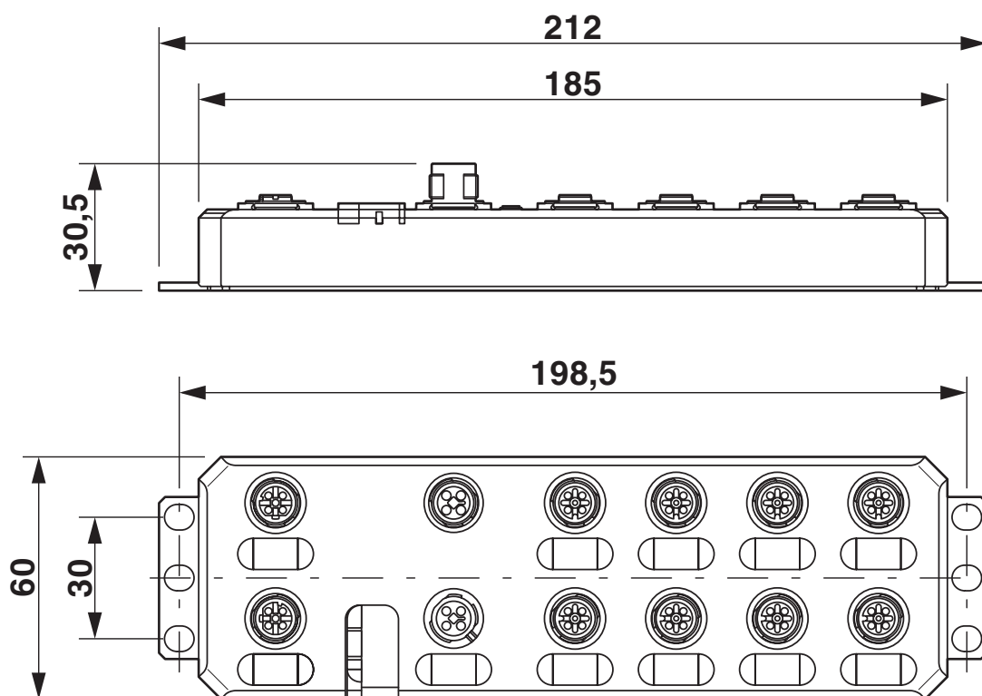
Rysunek wymiarowy
