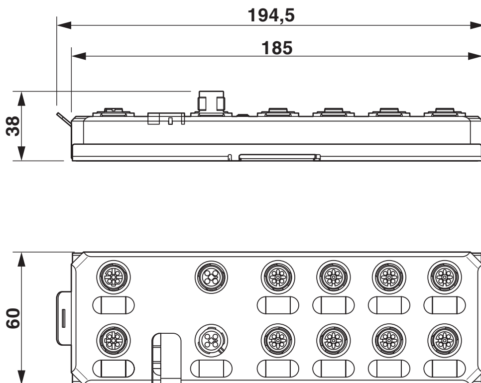
Rysunek wymiarowy
