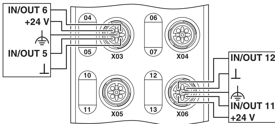
rysunek złączy
