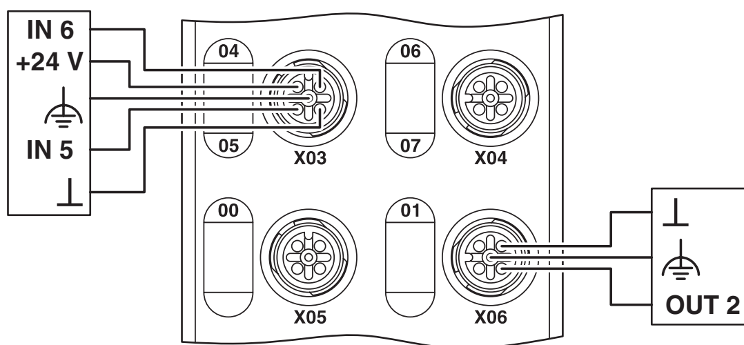
rysunek złączy
