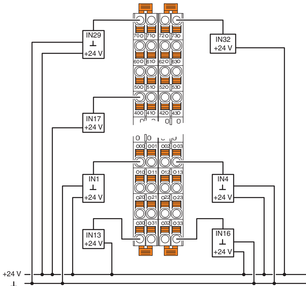
rysunek złączy
