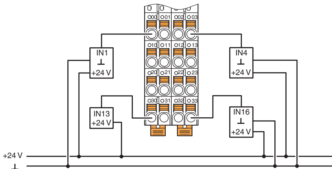
Przyłącze 1-przewodowe
