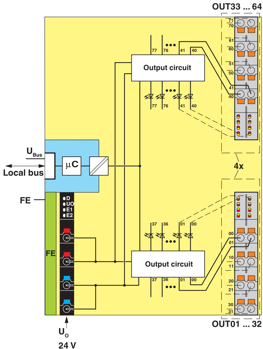
Schemat blokowy
