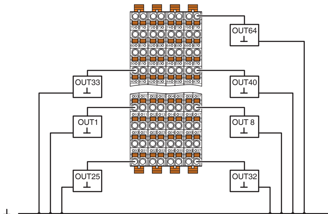
rysunek złączy
