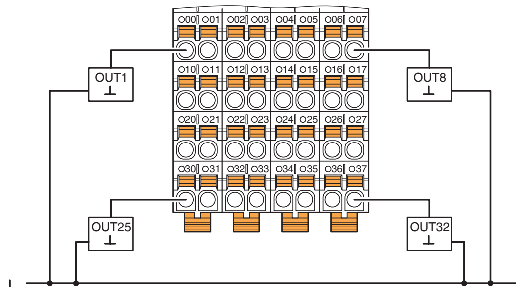
rysunek złączy
