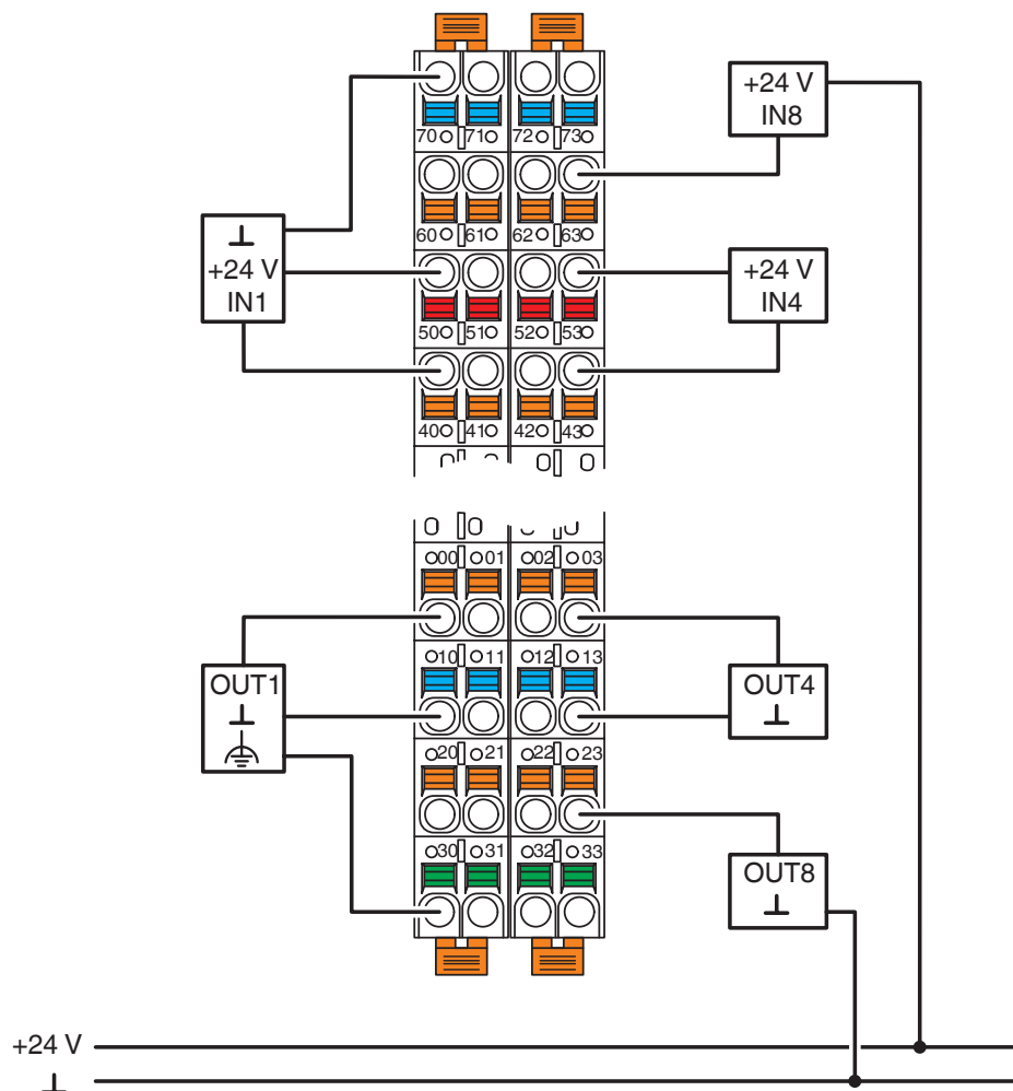
rysunek złączy
