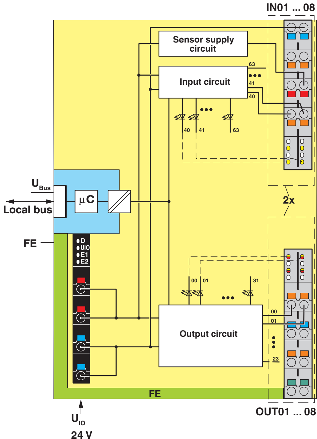
Schemat blokowy
