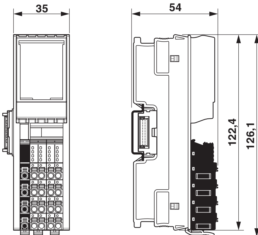
Rysunek wymiarowy
