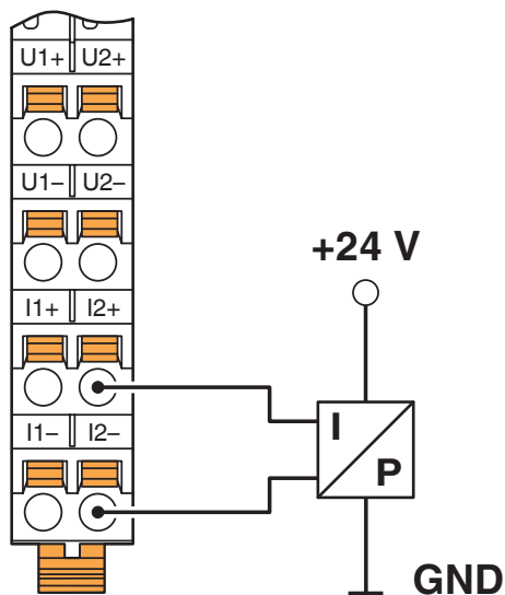
rysunek złączy
