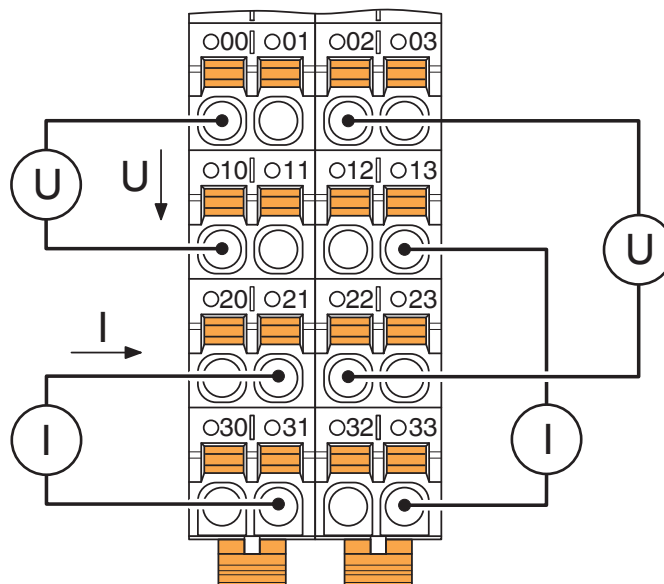
rysunek złączy
