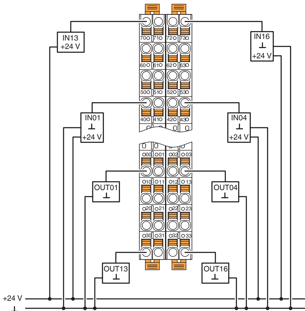
rysunek złączy
