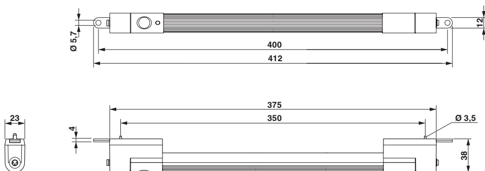
Rysunek wymiarowy
