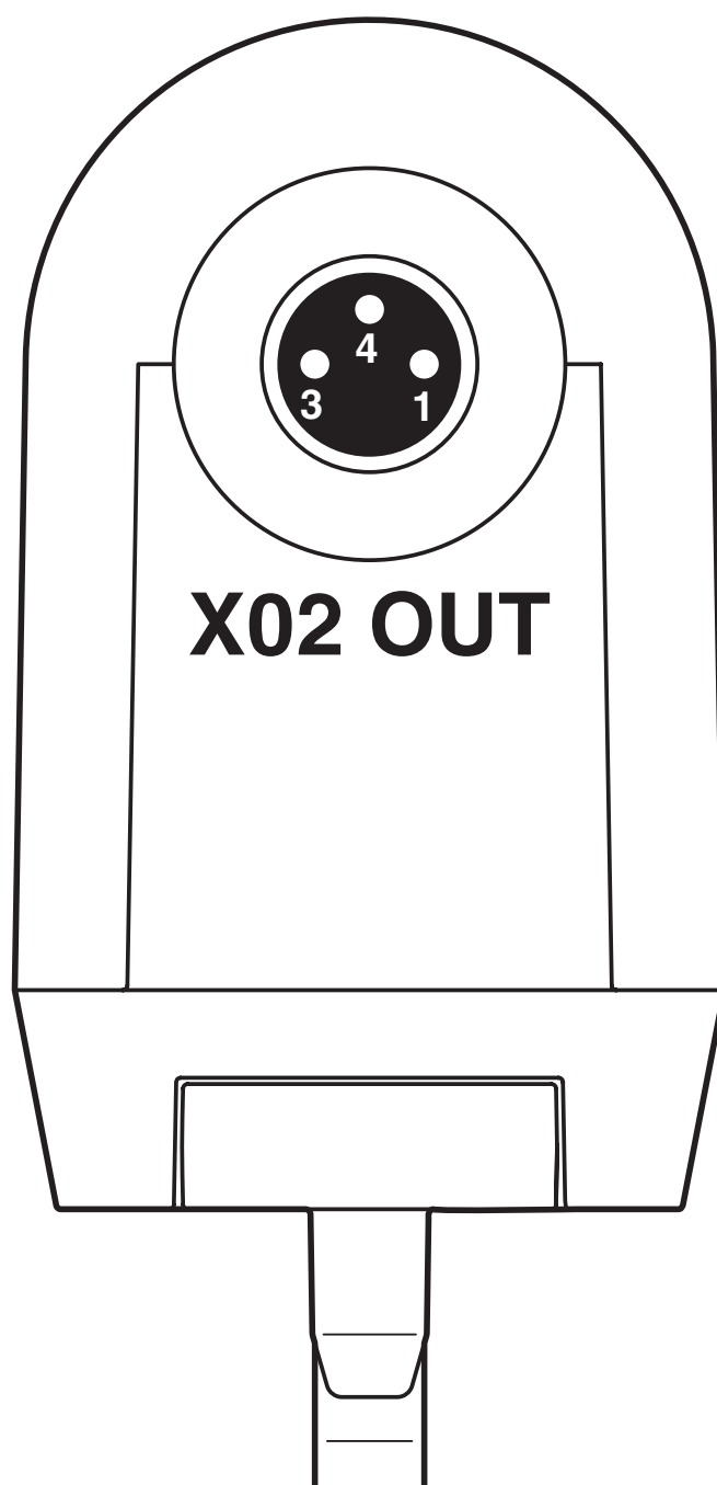
rysunek złączy
