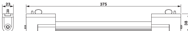
Rysunek wymiarowy
