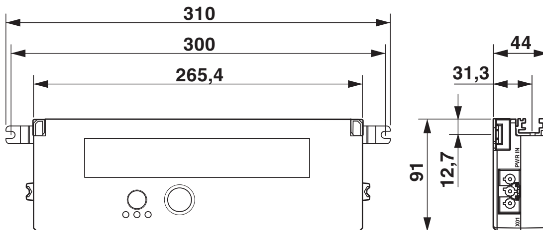
Rysunek z wymiarami do montażu przykręcanego
