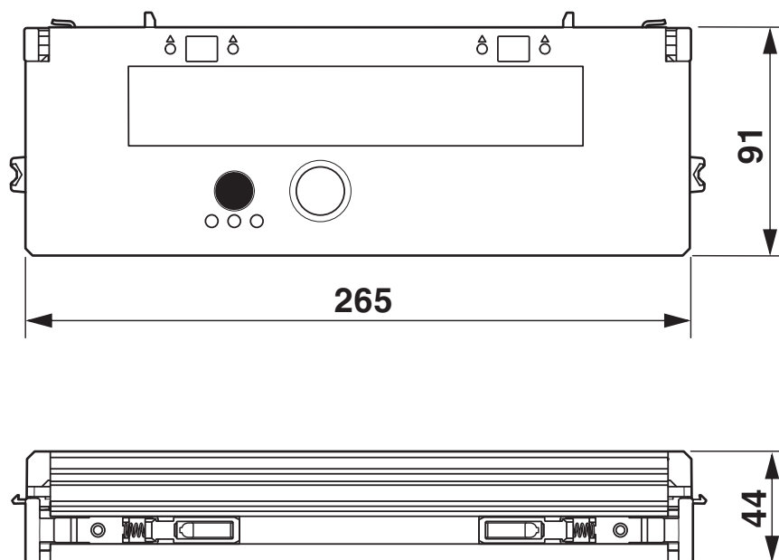
Rysunek wymiarowy
