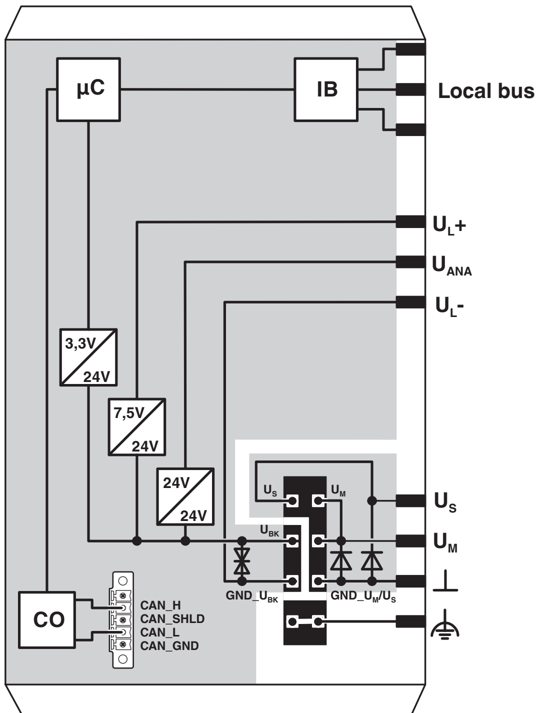
Schemat blokowy
