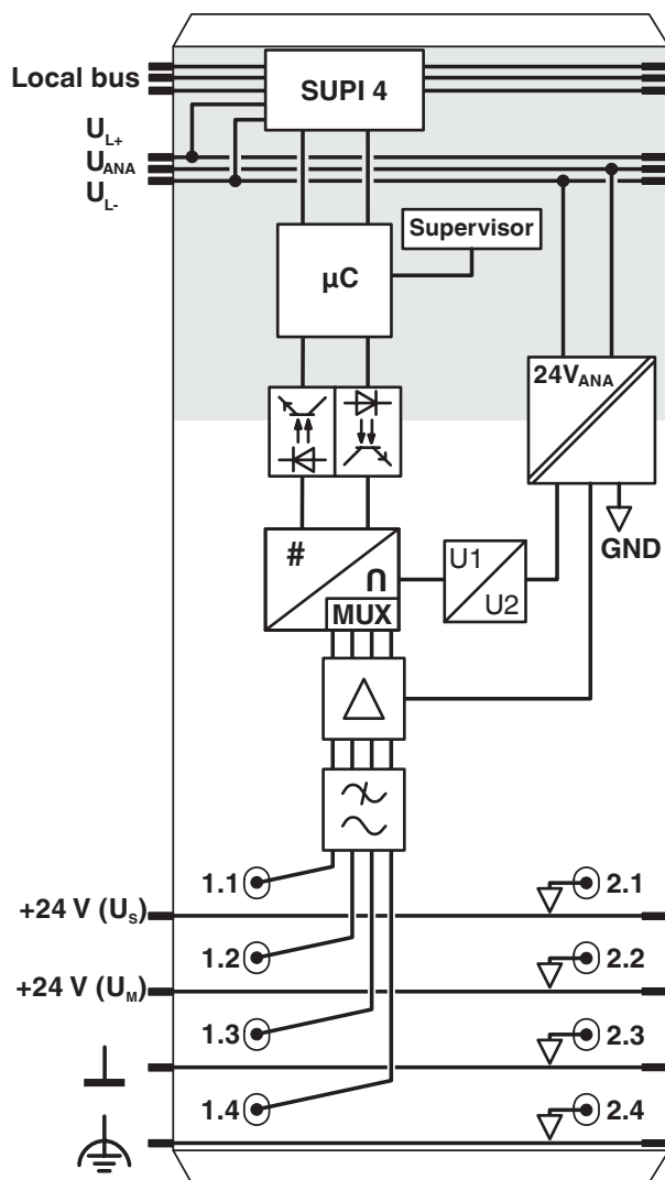
Schemat blokowy
