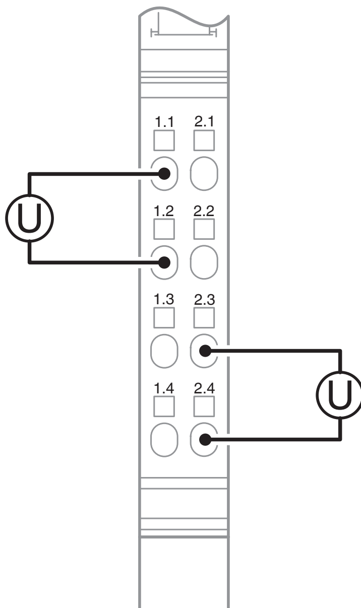
rysunek złączy
