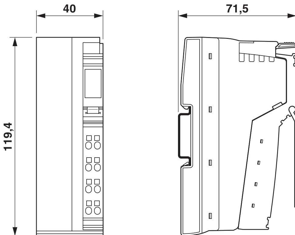
Rysunek wymiarowy
