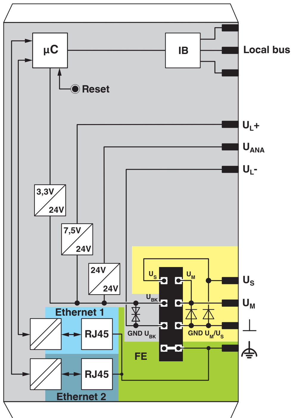
Schemat blokowy
