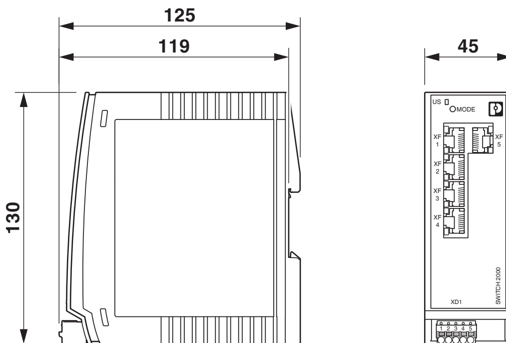
Rysunek wymiarowy
