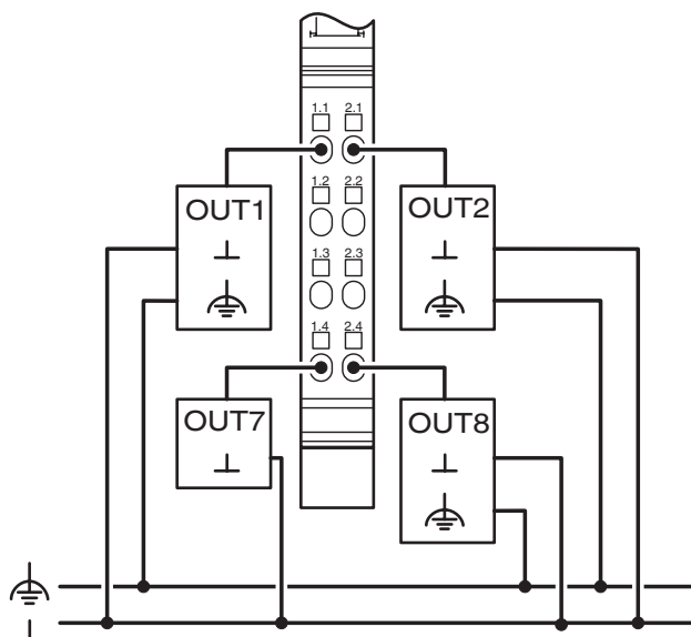
rysunek złączy
