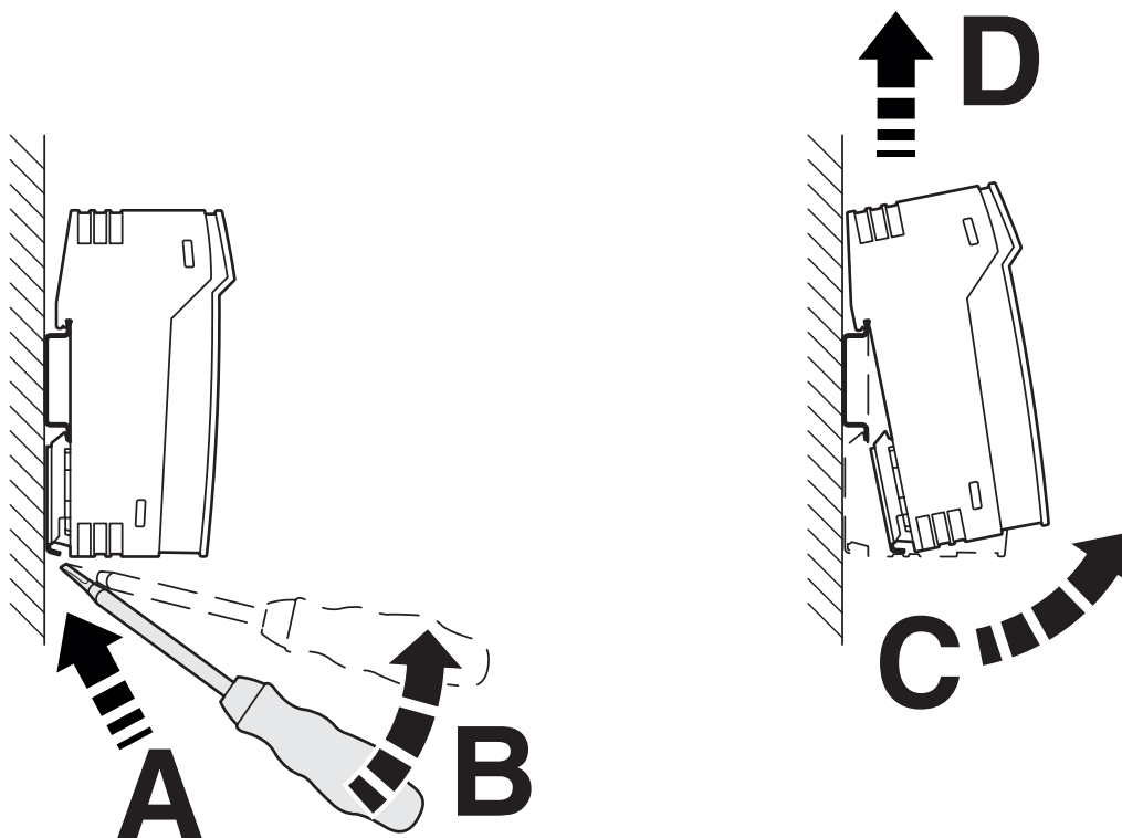
Rysunek schematyczny
