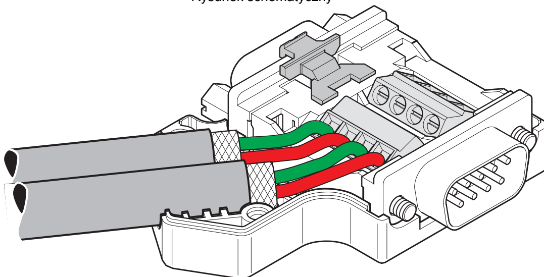
Rysunek schematyczny
