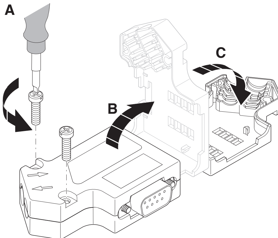
Rysunek schematyczny
