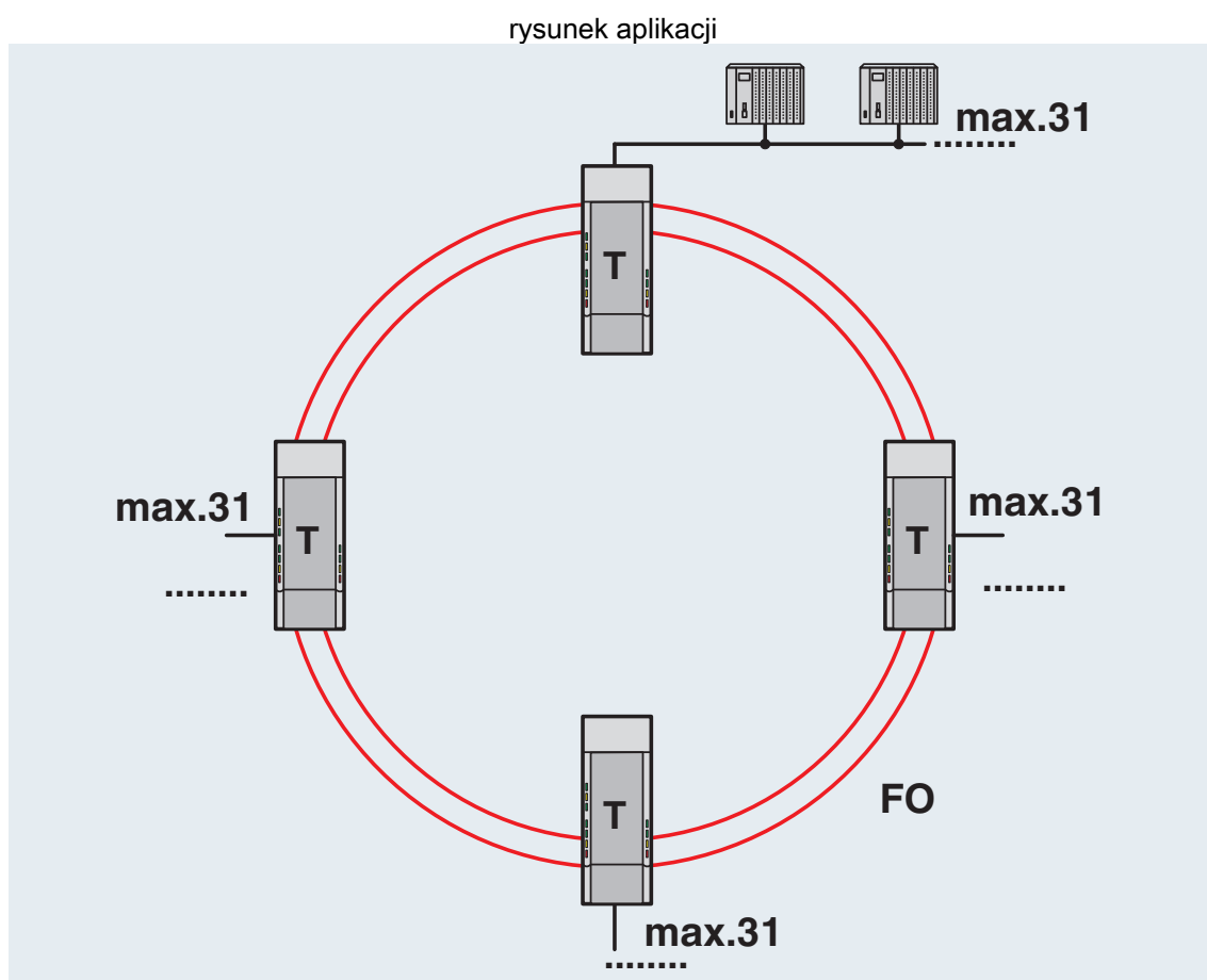
Redundantny pierścień światłowodowy
