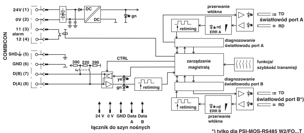
Schemat blokowy
