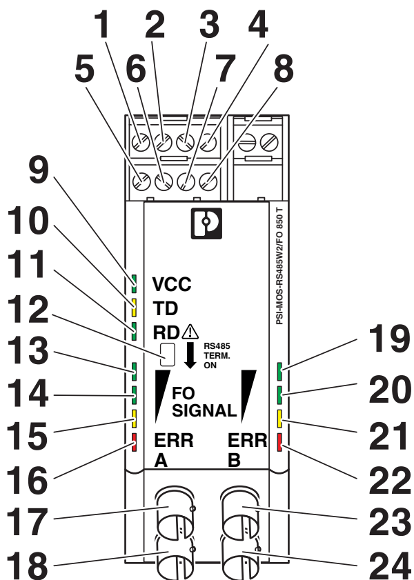
Rysunek schematyczny
