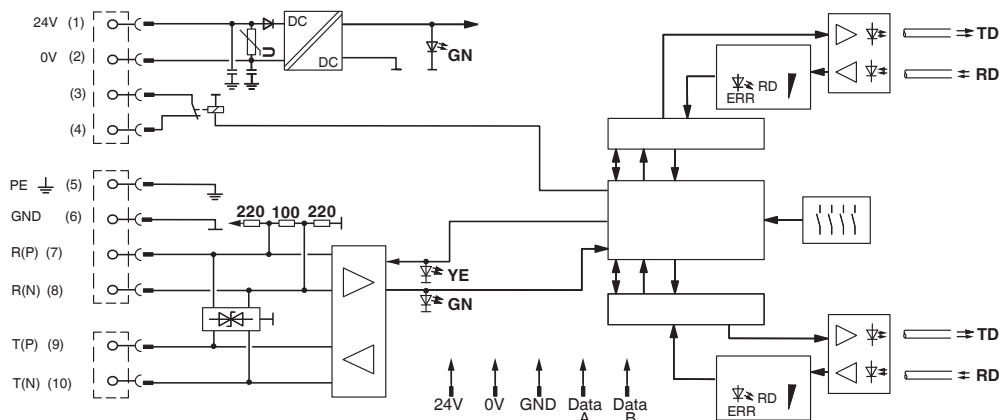
Schemat blokowy
