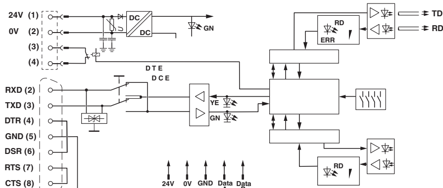
Schemat blokowy
