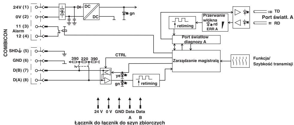
Schemat blokowy
