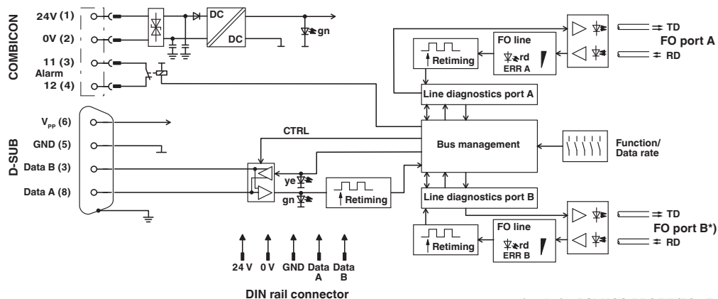
Schemat blokowy
