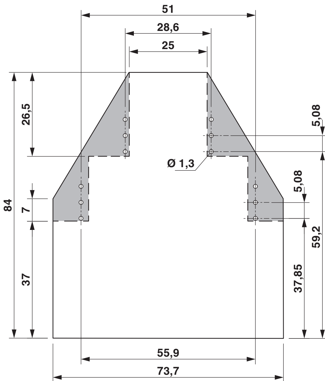
Rysunek wymiarowy
