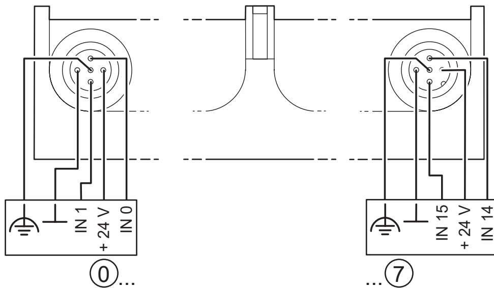
rysunek złączy
