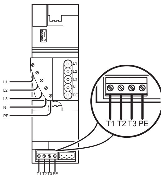
rysunek złączy
