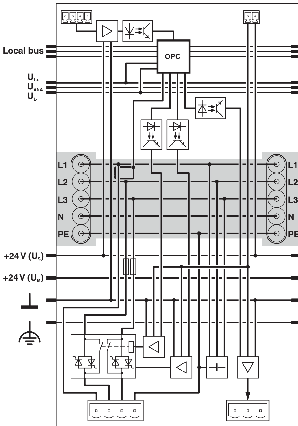
Schemat blokowy
