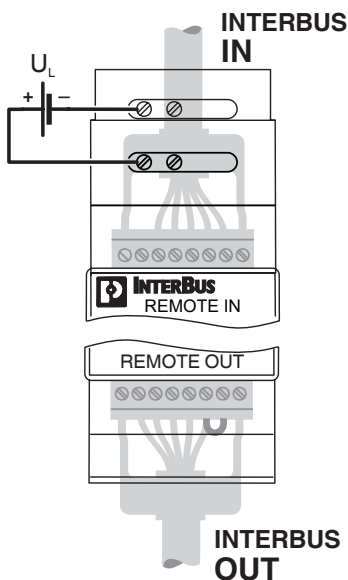
rysunek złączy
