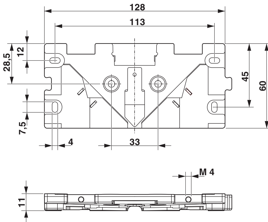
Rysunek wymiarowy
