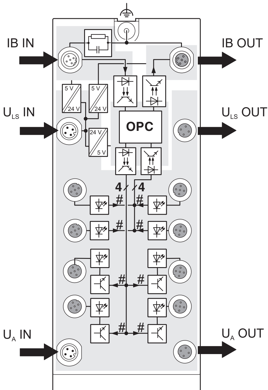
Schemat blokowy
