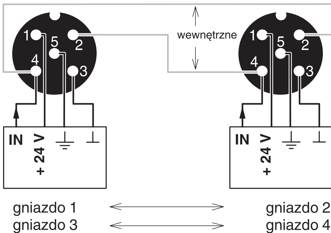
rysunek złączy
