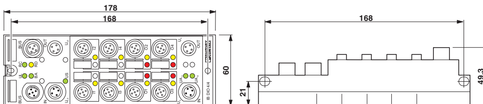
Rysunek wymiarowy
