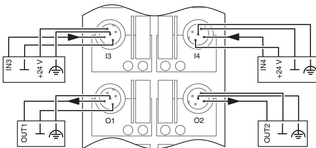
rysunek złączy
