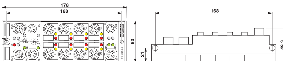
Rysunek wymiarowy
