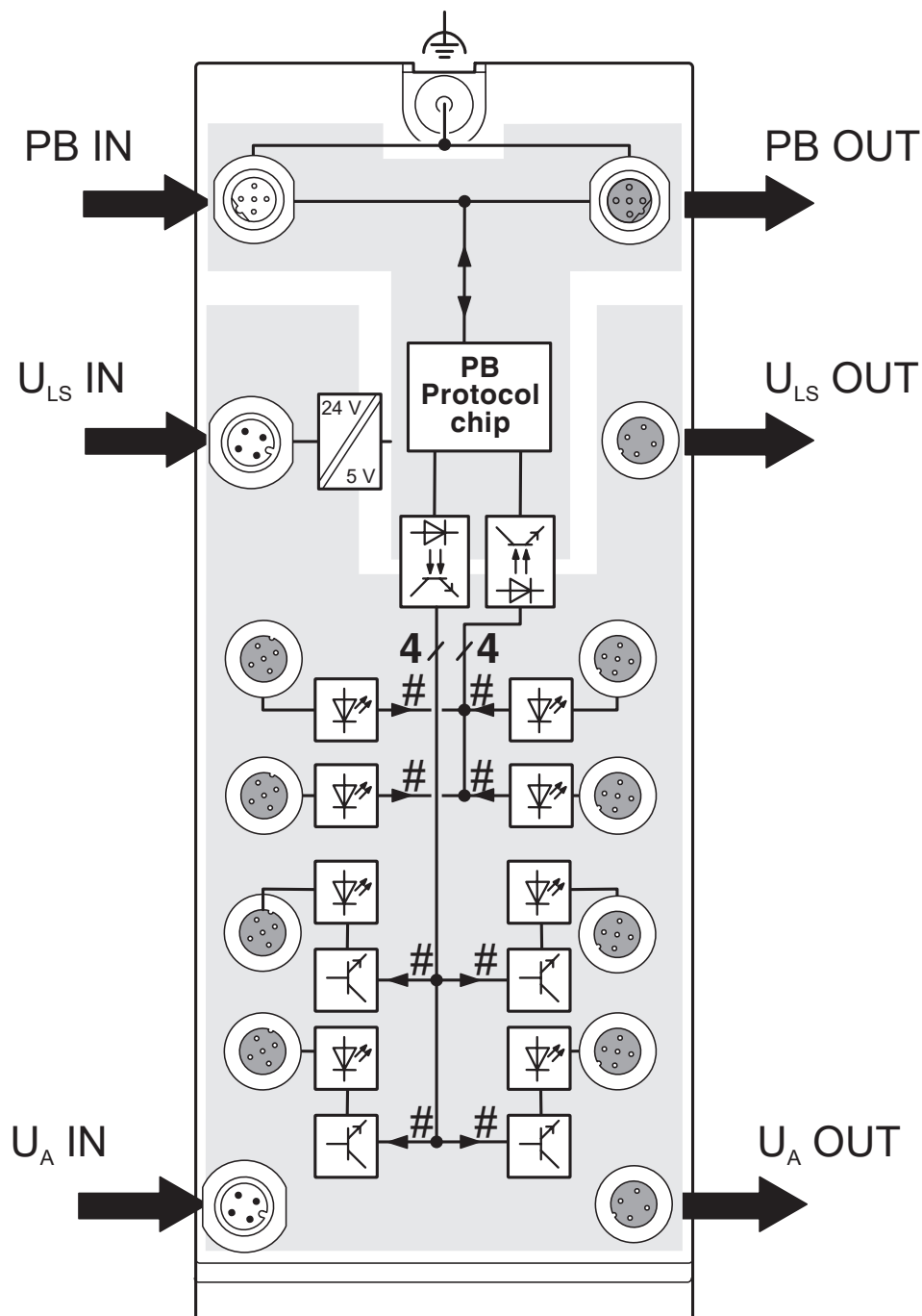
Schemat blokowy
