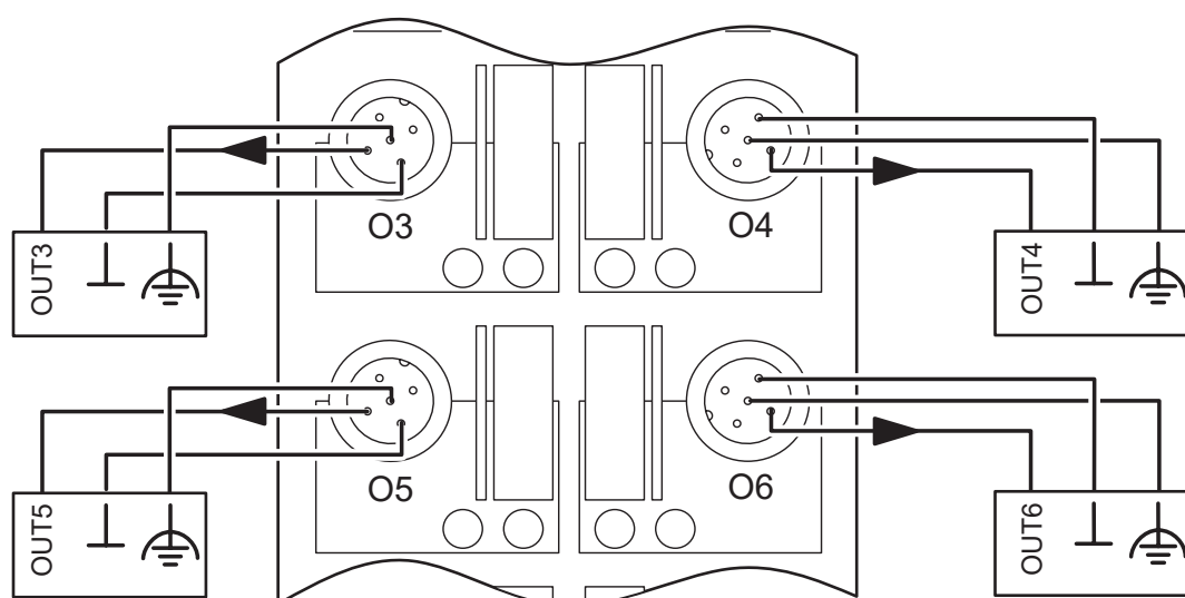
rysunek złączy
