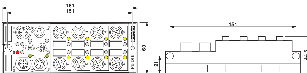
Rysunek wymiarowy
