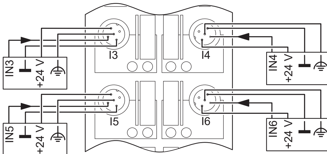
rysunek złączy
