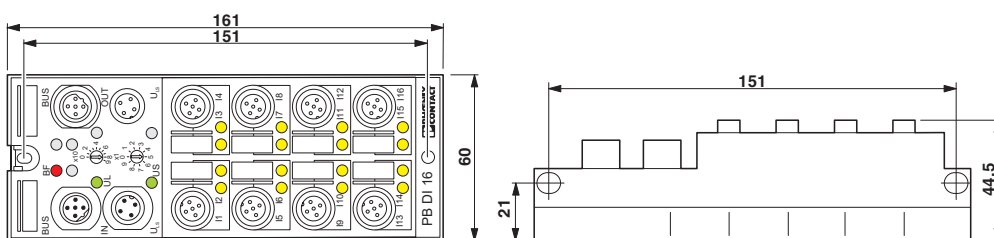
Rysunek wymiarowy
