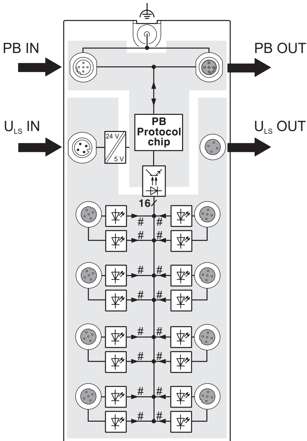
Schemat blokowy
