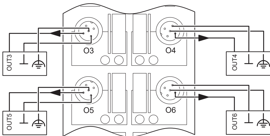
rysunek złączy
