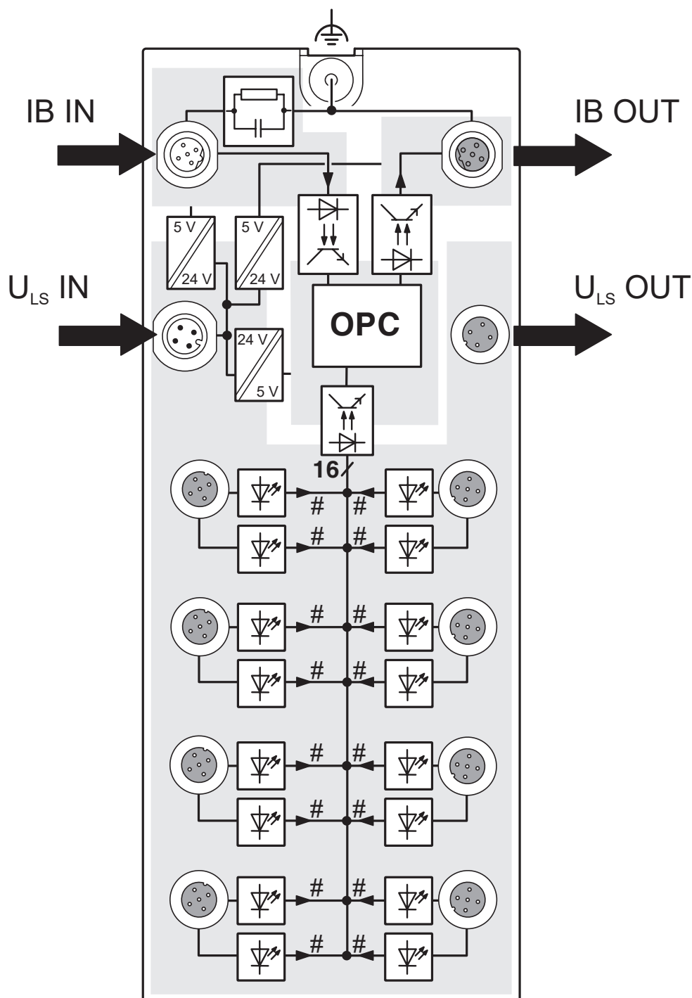
Schemat blokowy
