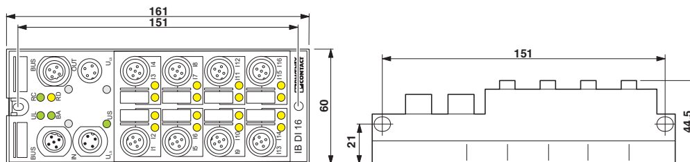
Rysunek wymiarowy
