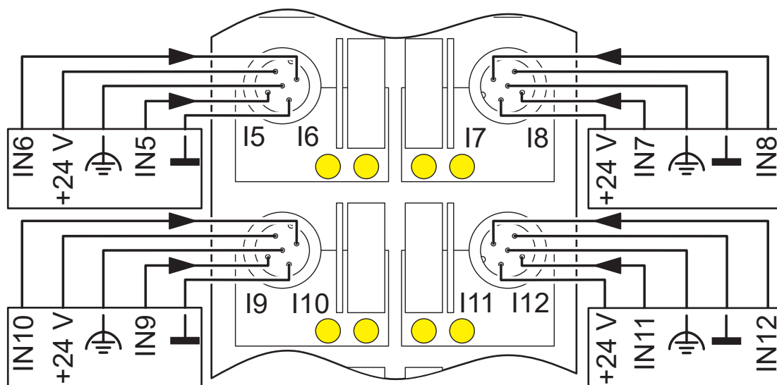
rysunek złączy
